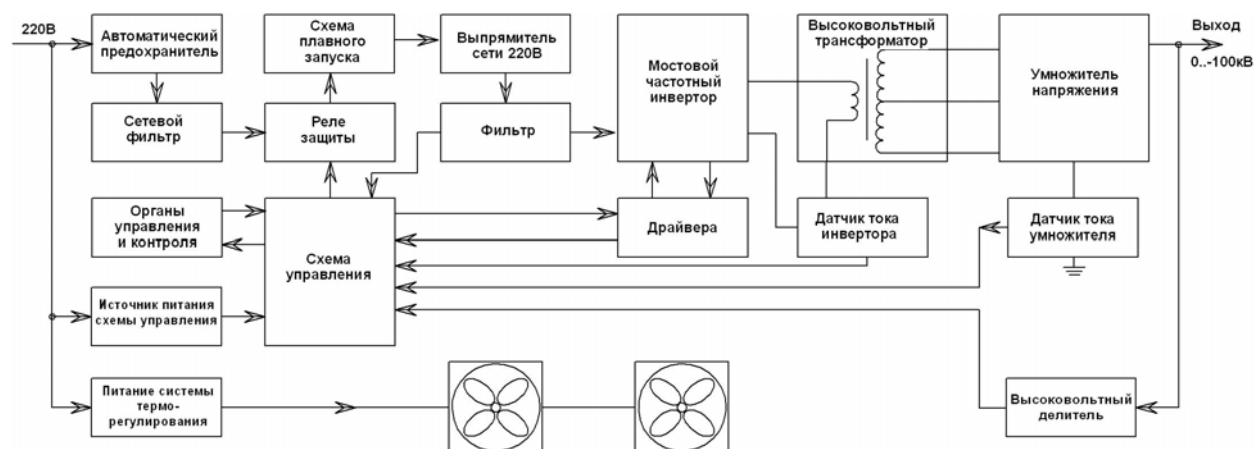
Рис. 4.1 Структурная схема зарядного устройства.
