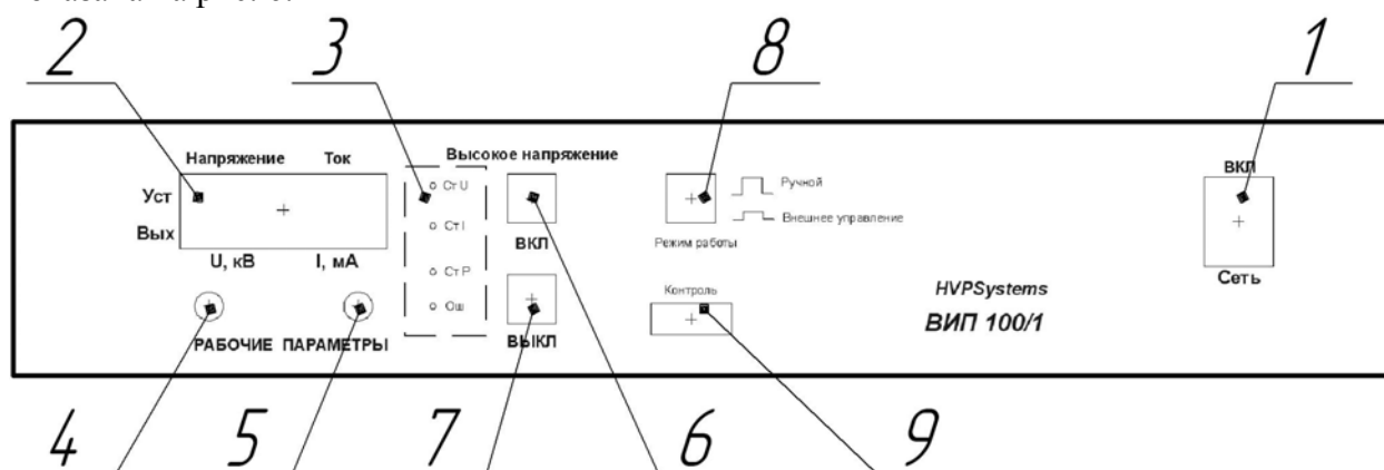
Рис. 6.1 Передняя панель прибора.
