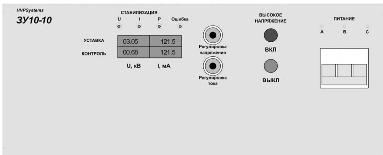
Рис. 5.1 Передняя панель ЗУ10-10.
